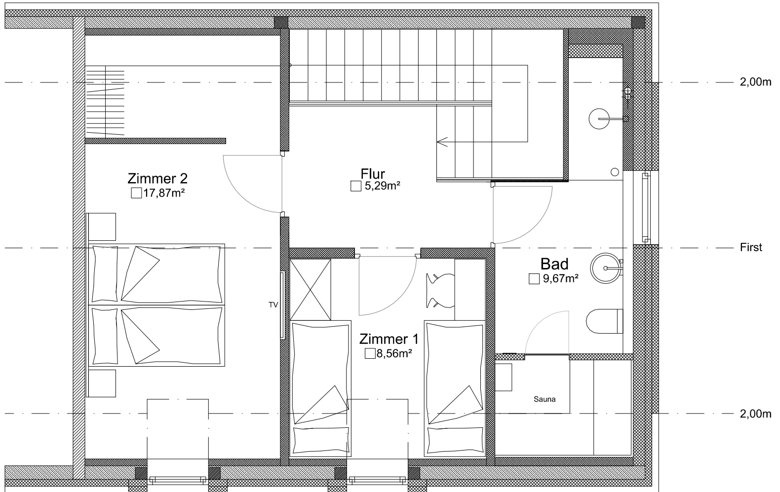
17 Anton Grundriss Obergeschoss
