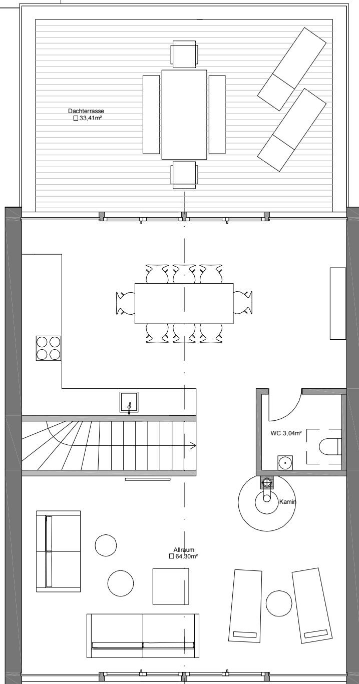
Grundriss Obergeschoss
