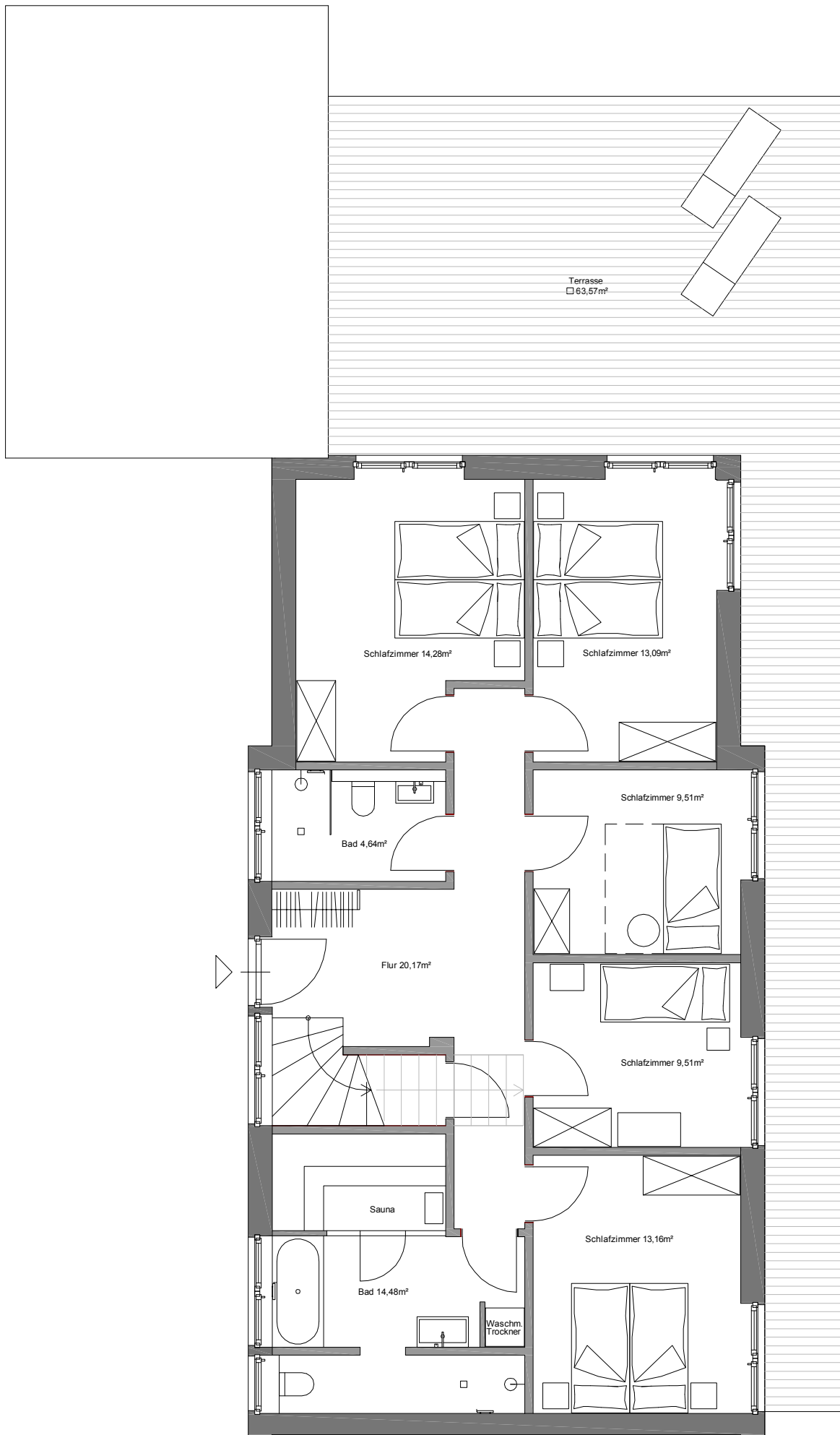
Grundriss Erdgeschoss
